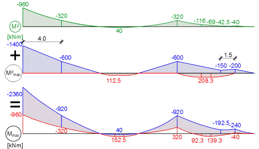
Statikailag határozott tartók maximális igénybevételi ábrái
