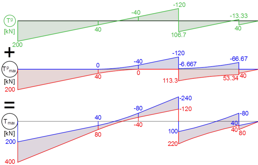
Statikailag határozott tartók maximális igénybevételi ábrái
