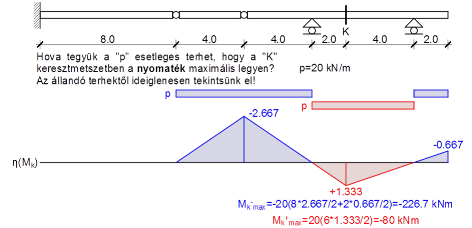
Statikailag határozott tartók maximális igénybevételi ábrái
