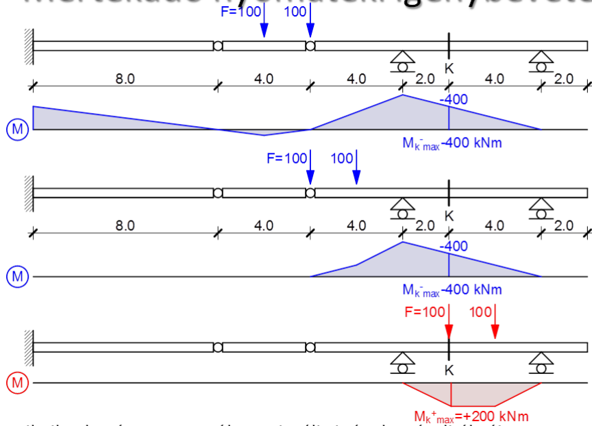
Statikailag határozott tartók maximális igénybevételi ábrái
