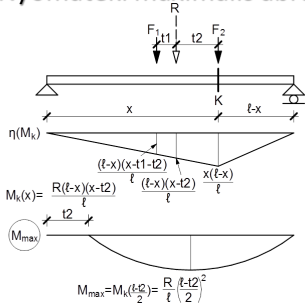
Statikailag határozott tartók maximális igénybevételi ábrái
