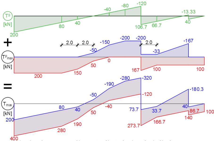
Statikailag határozott tartók maximális igénybevételi ábrái
