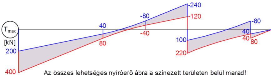
Statikailag határozott tartók maximális igénybevételi ábrái
