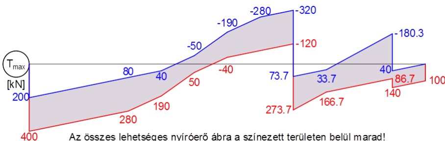
Az összes lehetséges nyíróerő ábra a színezett területen belül marad! Statikailag határozott tartók maximális igénybevételi ábrái
